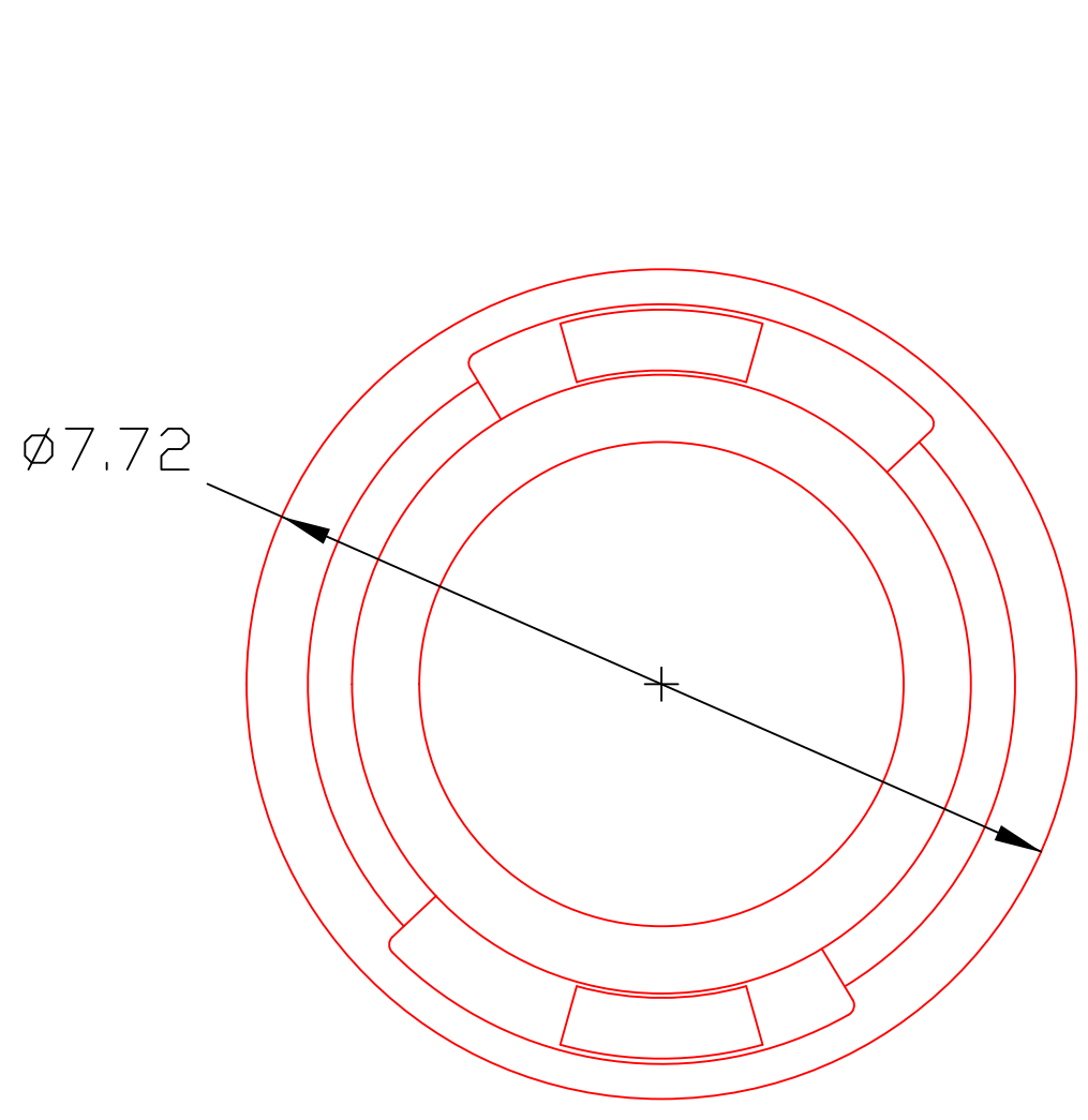
5" STORZ
